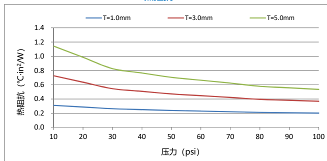
热阻抗
